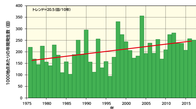
全国(アメダス)の1時間降水量50mm以上の年間発生回数の経年変化(1976~2017年)
